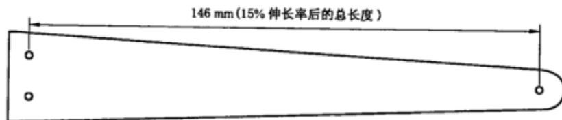
图5 用于将试样安装在试样架上时确定两端孔距的模板
