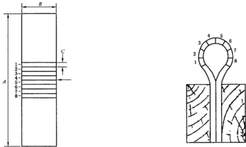
A——试样长度,95 mm; B——试样宽度,(25±0.5)mm; C——由试样中部平行线开始往两端的画线,每两条平行画线之间的距离,3.2 mm。
